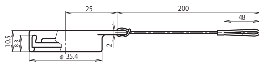
アダプタゴムキャップ：NRW-28-AdCa
