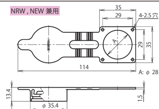
レセプトクルゴムキャップ：NRW-28-RCa・2
