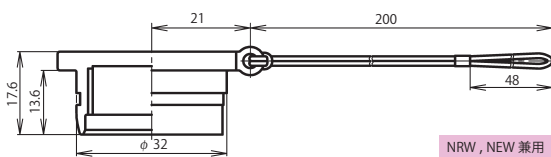
プラグ防水キャップ：NRW-28-PCa・1
