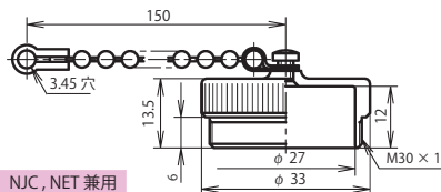
プラグキャップ：NJC-28-PCa
