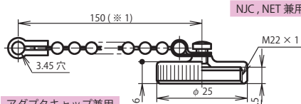
レセプタクルキャップ：NJC-20-RCa
